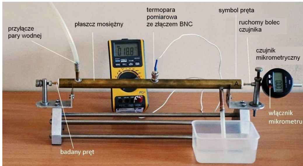
Rys. 1. Dylatometr - przyrząd do mierzenia współczynnika rozszerzalności cieplnej ciała
