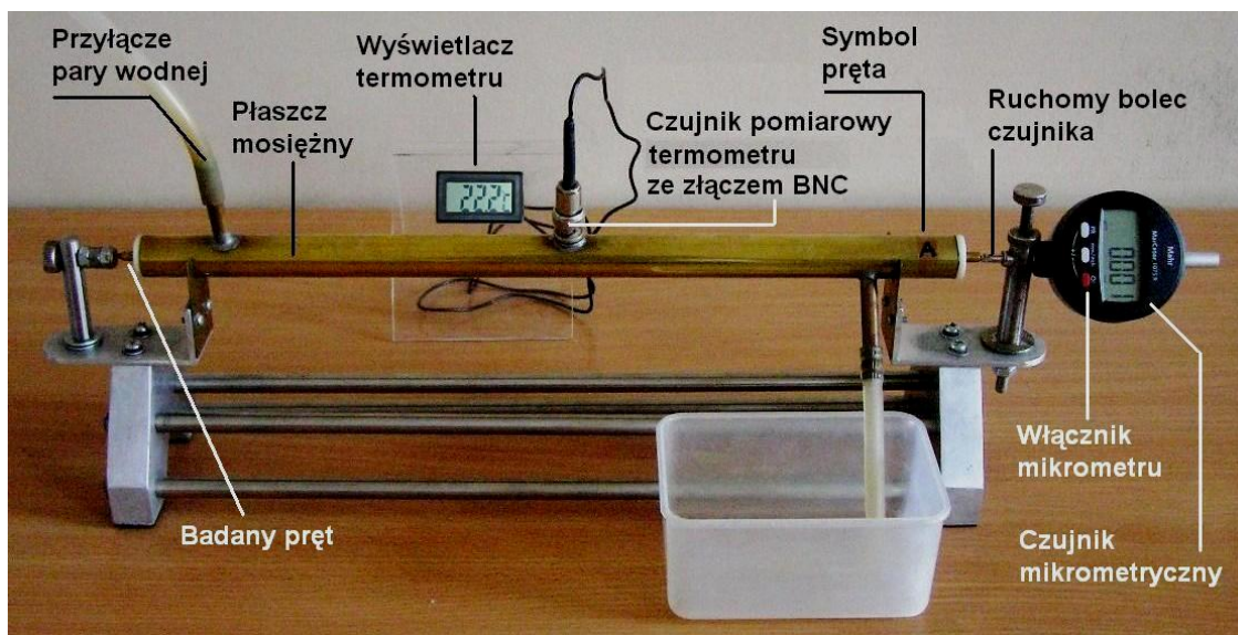
Rys. 1. Dylatometr - przyrząd do mierzenia współczynnika rozszerzalności cieplnej ciała
