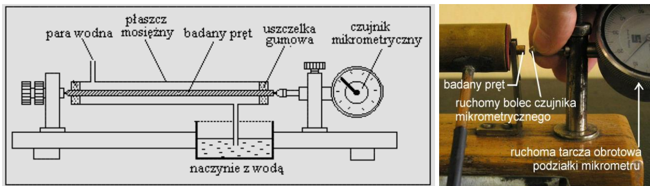
Rys. 8. Dylatometr z mikrometrem analogowym - przyrząd do mierzenia współczynnika rozszerzalności cieplnej ciała.
