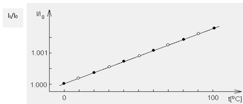
Rys. 6. Zależność l_t/l_0 od temperatury t wyznaczona dla ciał z rys. 5
